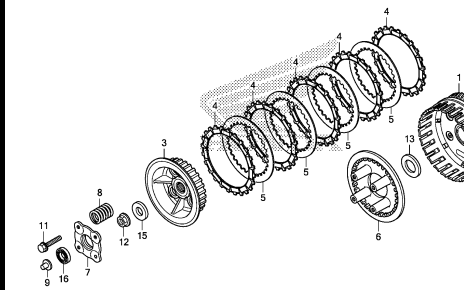
CLUTCH
