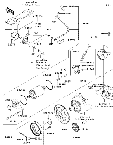
23 Starter Motor - มอเตอร์สตาร์ท
