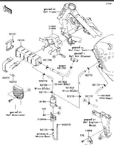
19 Fuel Evaporative System - ระบบควบคุมไอน้ำมันเชื้อเพลิง
