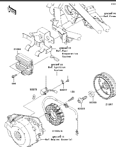
21 Generator - แม่กนิต
