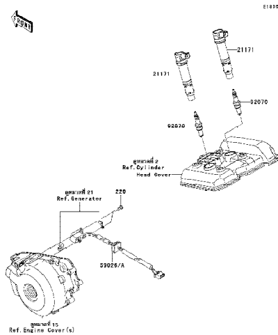
22 | Ignition System - คอยล์หัวเทียน
