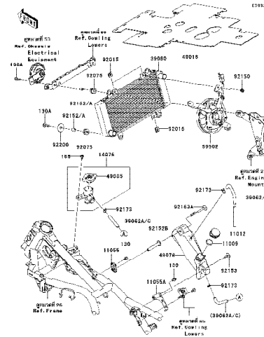
24 | Radiator - หม้อน้ำ
