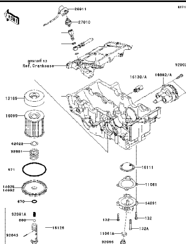
20 Oil Pump - ปั๊มน้ำมันเครื่อง
